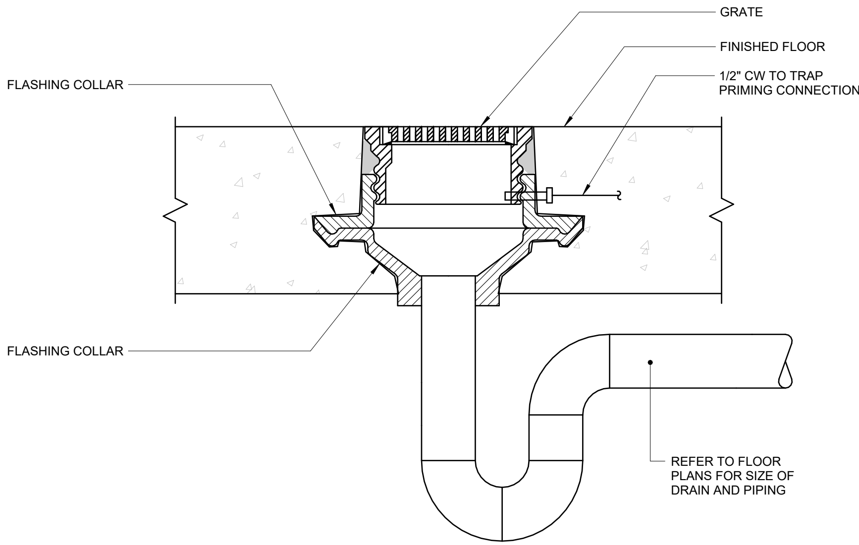
1 DETAIL - FLOOR DRAIN (TRAP PRIMER) SCALE: N.T.S.
